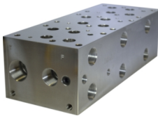
Block Manifold CETOP 8 Daman Presión Máx. (PSI):3000 Aluminio
